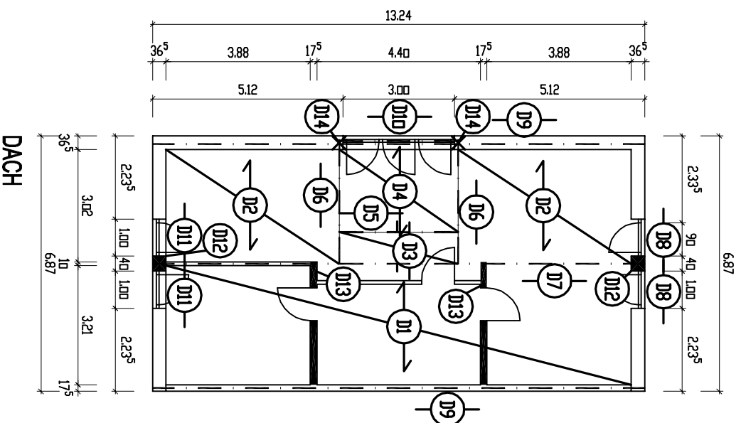
POSITIONSPLAN DACH
