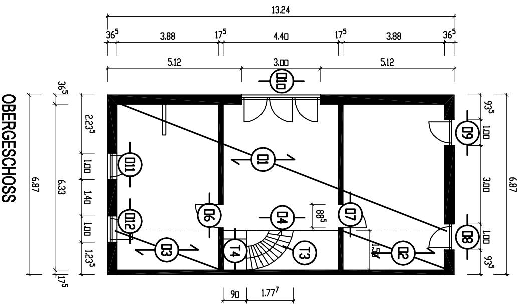
POSITIONSPLAN OG
